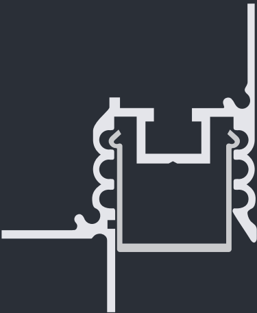
607C Scretto 49.6 x 60 mm
