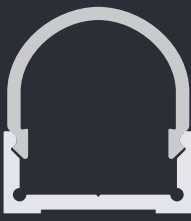
300C (-2B04) Doppio Tondo 25x28 25.4 x 28 mm
