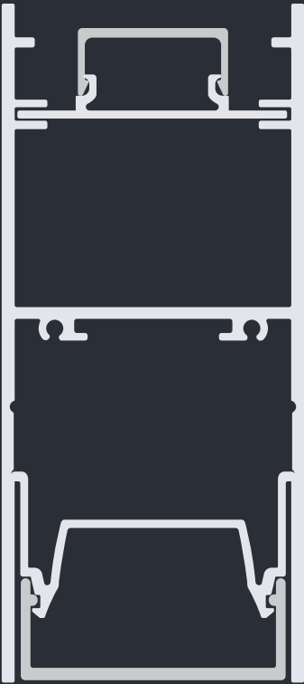
759E Modulo 44.7 x 100 mm
