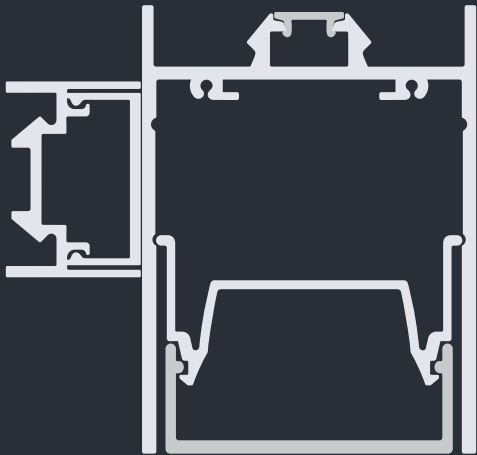
7565 Rigoletto 63.1 x 60 mm
