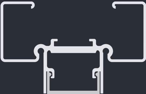
7C38 Montante Soffitto Luce a filo 65 x 41 mm
