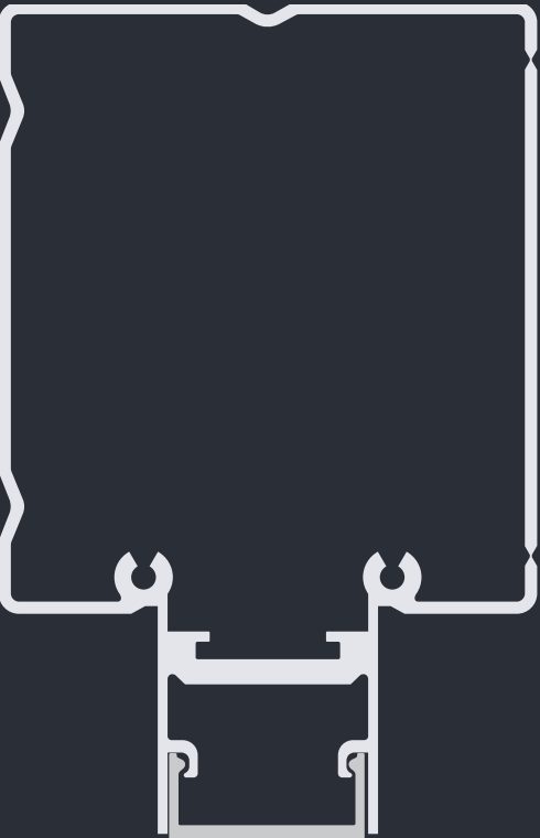
7C42 Montante Parete Luce a filo parete 65 x 100.3 mm
