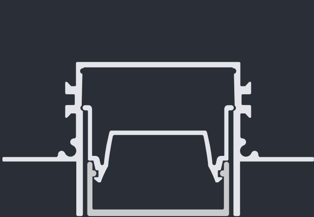
76C0 Incasso Modulo 84.6 x 42 mm
