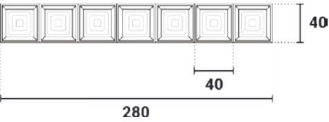
Sezione (mm) / Section (mm)
