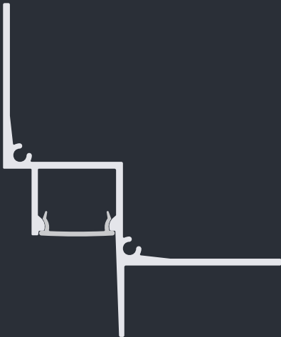
7C7E Gola di Luce 72.4 x 34 mm
