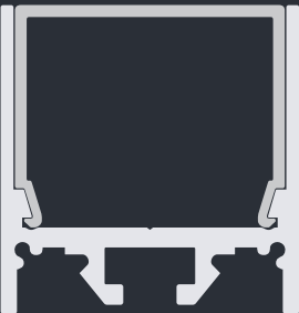
30D4 Ever 40x40 36 x 37 mm
