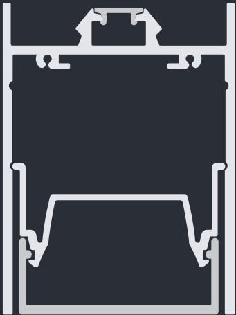
765C Modulo Mini 44.7 x 60 mm
