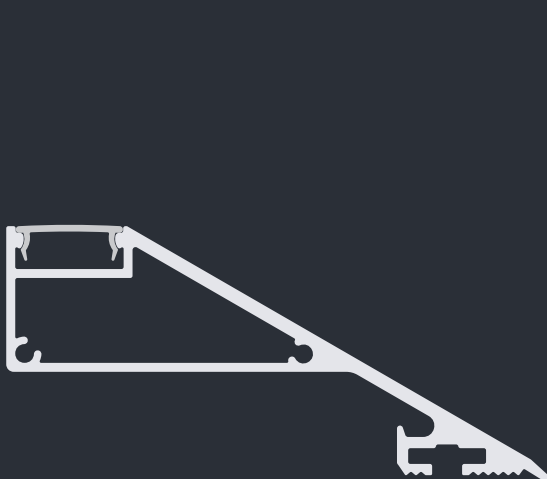
7C88 Profilo Edge 72.4 x 34 mm
