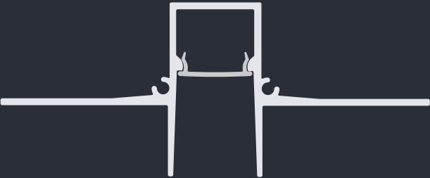
7CF6 Lama di Luce 81.4 x 33.1 mm
