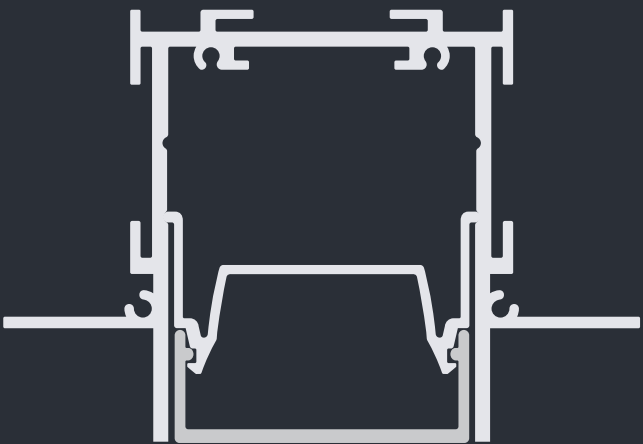
76D4 Incasso Modulo Alto 84.6 x 57.3 mm
